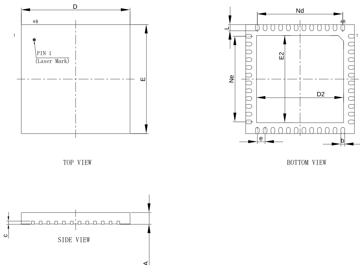
图 25 QFN48 封装图
