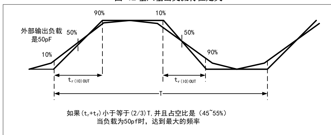
图 12 输入输出交流特性定义
