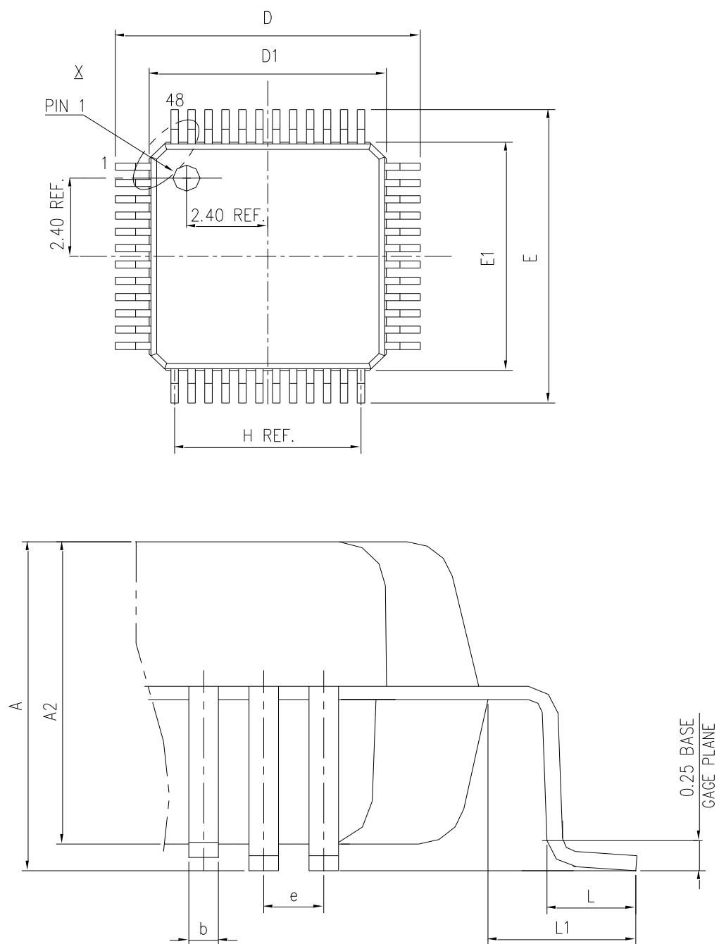
图 20 LQFP48 封装图
